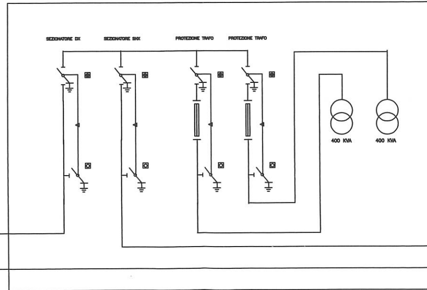
CABINA UFFICI
